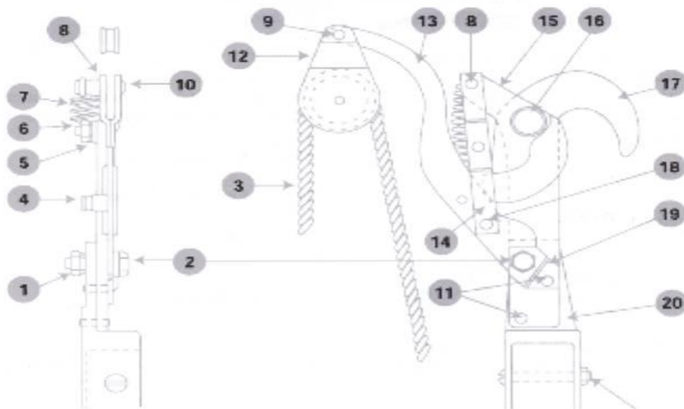
Pièces pour tête «Marvin»
